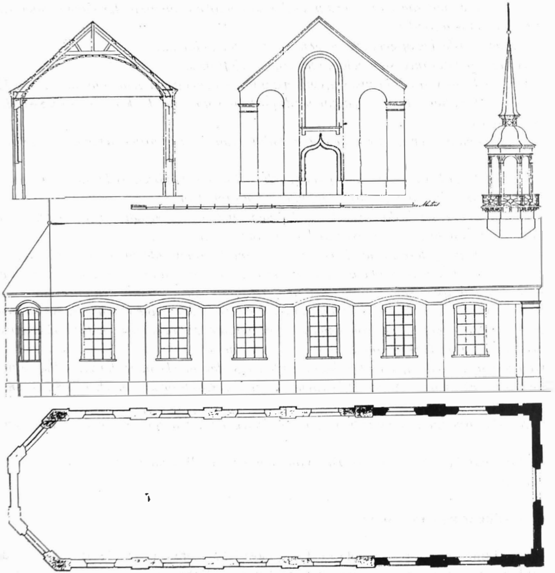
20. Afgekeurd plan verlenging kerk Overslag (1850). RAG Provinciaal archief, 1851-1870, nr. 1823.
